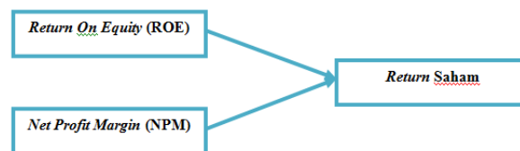
Gambar 1. Kerangka Konseptual
