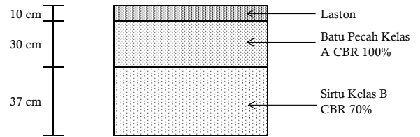
Gambar 4.1 Susunan Perkerasan
