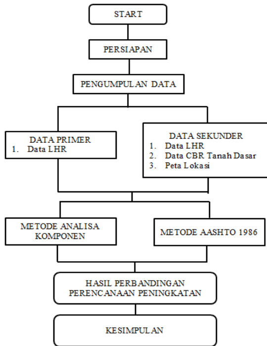
Gambar 3.2 Bagan Alir Perencanaan (Flowchart) Peningkatan Jalan
